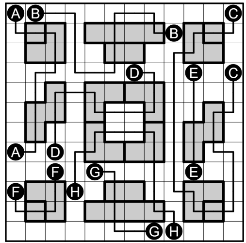
4.8 Arukone POM
