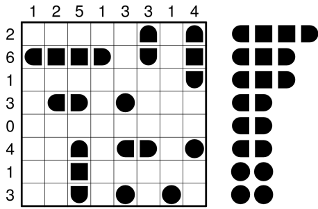
5.7 Schiffe Versenken
