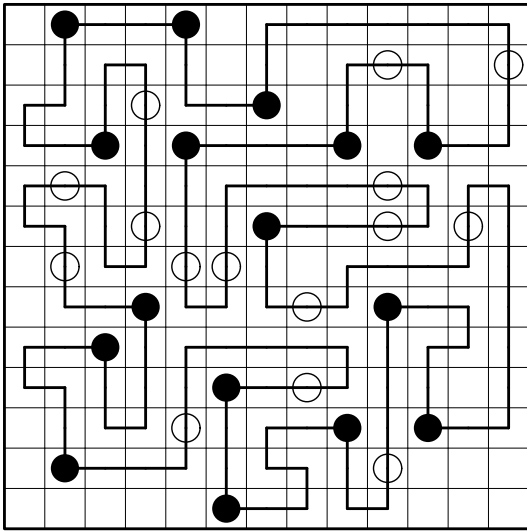
4.1 Masyu
