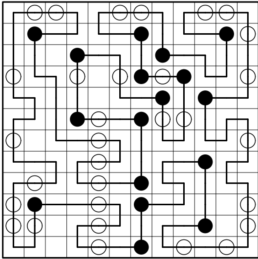
4.7 Masyu-Rekonstruktion
