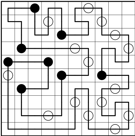
4.3 Variables Masyu
