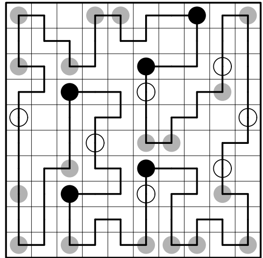
4.4 Graues Masyu
