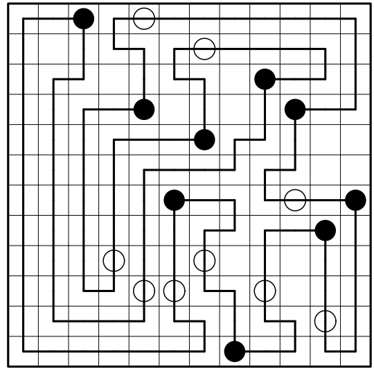
4.2 Alternierendes Masyu
