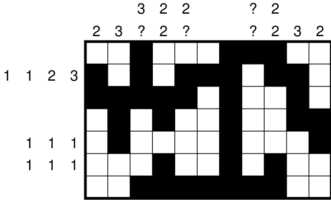
2.1 Koralle
