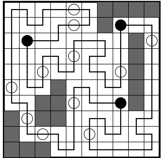
2.4 Pentomino-Masyu
