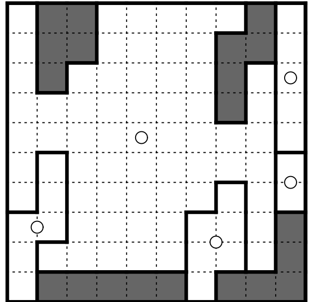
2.5 Pentomino-Galaxien
