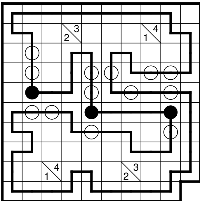
2.3 Tapasyu
