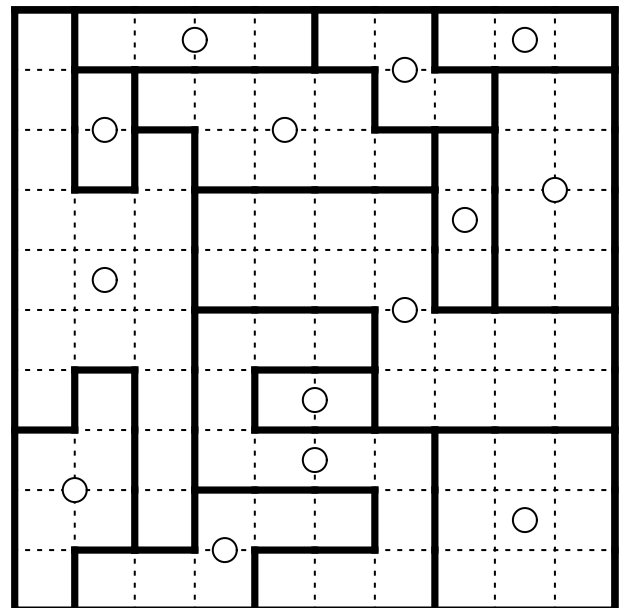
2.6 Galaxien
